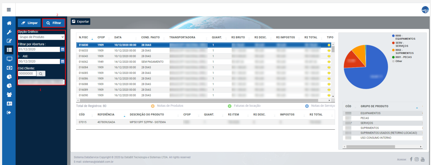
Figura 41 - Gráfico Notas
