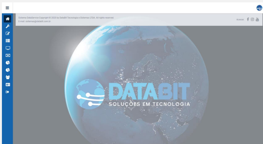
Figura 2 – Tela Inicial
