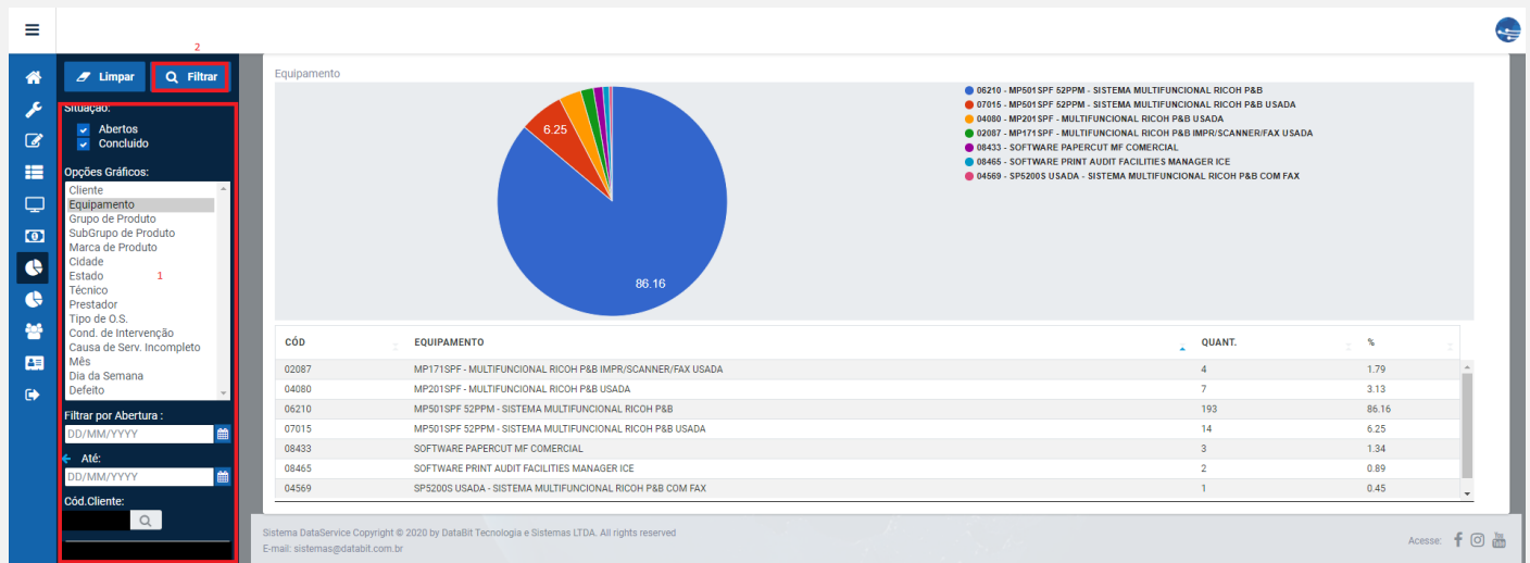
Figura 54 - Gráfico OS
