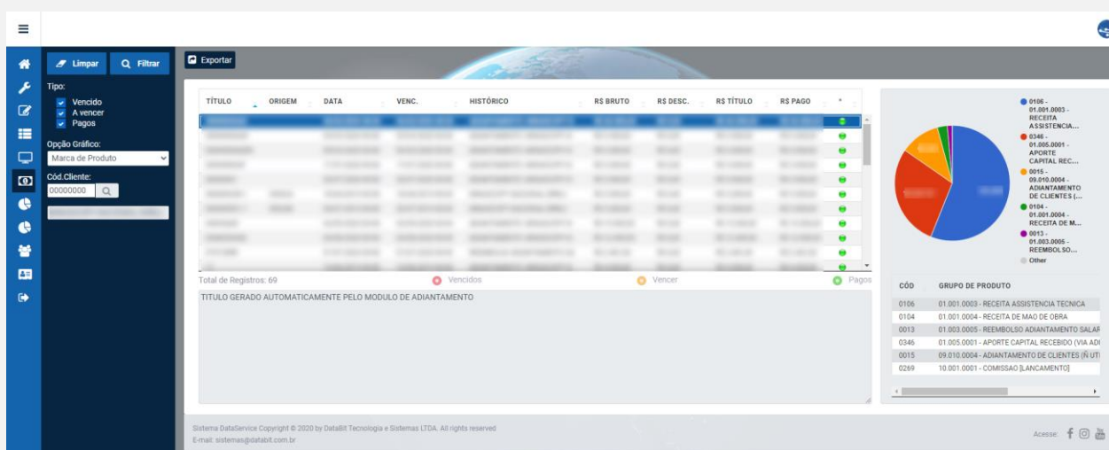
Figura 50 - Gráfico Financeiro
